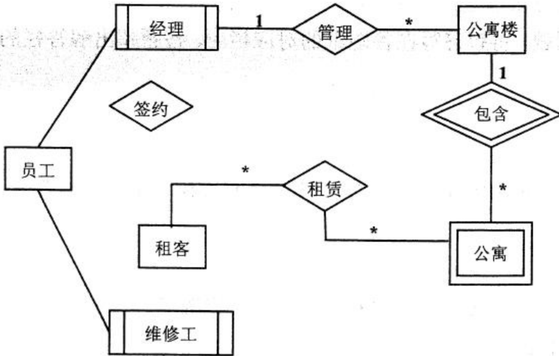
图 2-1 实体联系图
