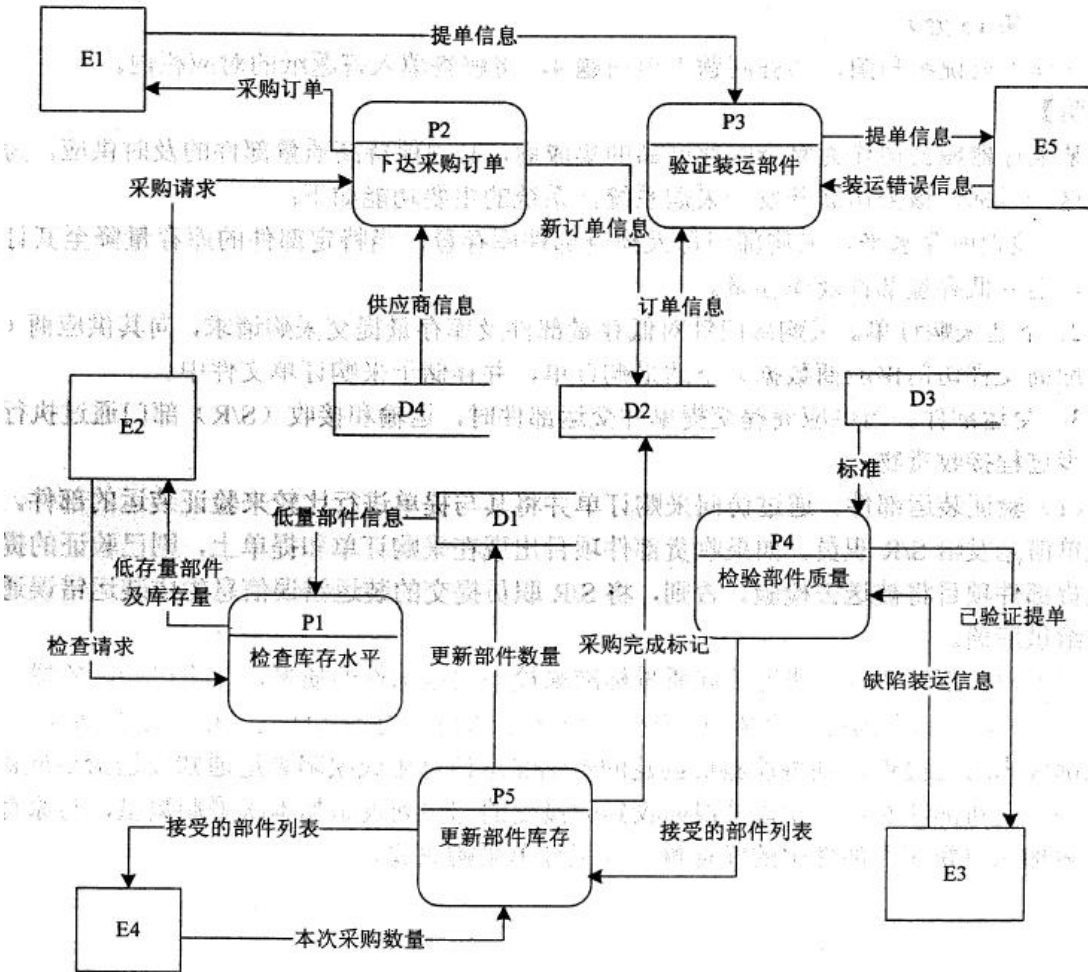
图 1-2 0层数据流图
