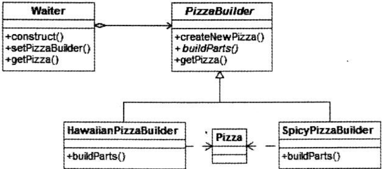
图 5-1 类图
