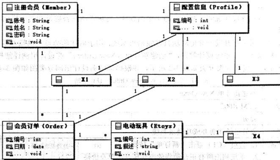
图 3-1 部分类图
